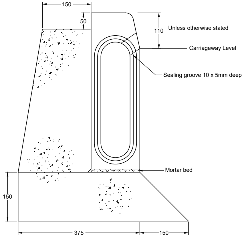
End Elevation
